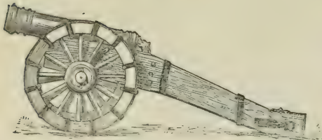
( محاصره طوبی )
